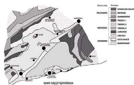
Mapa geològic esquemàtic del Penedès i Garraf (a dalt) i Principals relleus i estructures geològiques del Penedès i Garraf (a la dreta)
