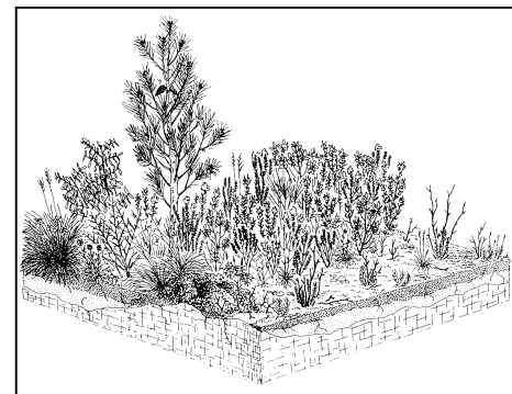
Esquema de la brolla de romaní i bruc d'hivern.
