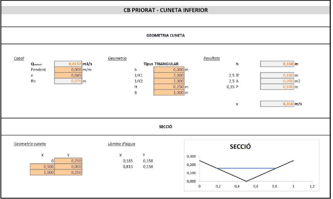
Figura 6. Càlculs de comprovació de la capacitat de la cuneta
