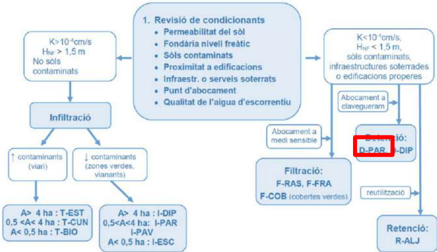
Figura 3. Diagrama de flux per la selecció de la tipologia de SUDS.
