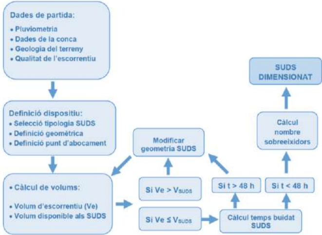
Figura 4. Passos a seguir pel dimensionament dels SUDS.
